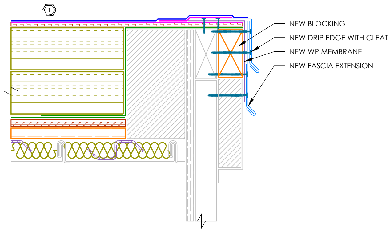
1 RAKE EDGE NTS
